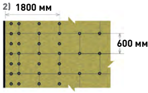
Рис. 7.8. Схема установки связей 1) в основном поле стены, 2) в углу здания в системе слоистой кладки
