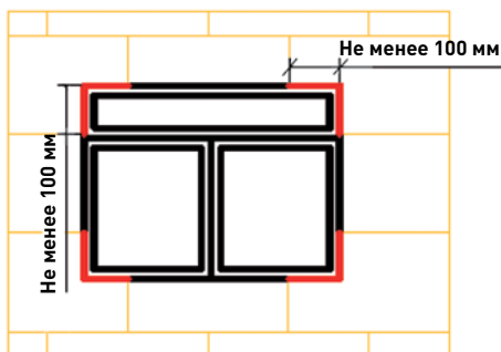
Рис. 7.26. Укладка плит вокруг оконных и дверных проемов
