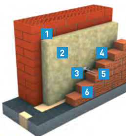
Рис. 7.7. Система ТН-ФАСАД Стандарт
