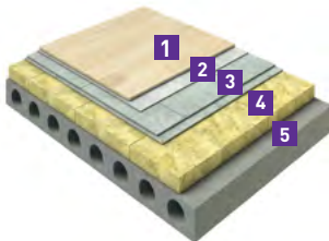
Рис. 5.8. Система ТН-ПОЛ Проф
