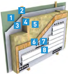
Рис. 7.13. Система ТН-ФАСАД Эконом
