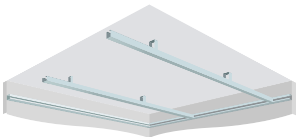
Рис. 5.15. Установка подвесов и потолочного профиля
