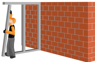
Рис. 6.3. Установка стоечного профиля
