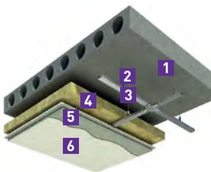
Рис. 5.12. Система ТН-ПОТОЛОК Акустик
