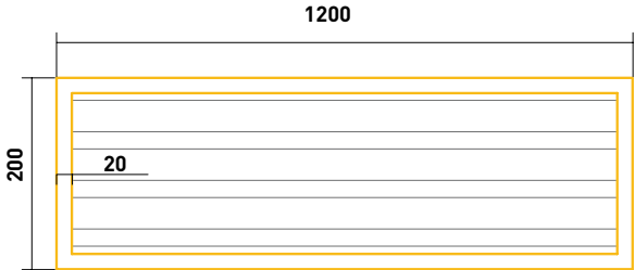
Рис. 7.22. Схема нанесения клея сплошным методом
