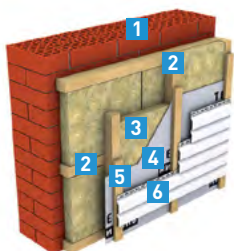
Рис. 7.1. Система ТН-ФАСАД Сайдинг
