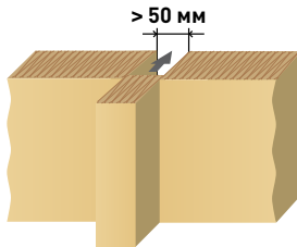
Рис.1.7. Плотное прилегание теплоизоляции при монтаже
