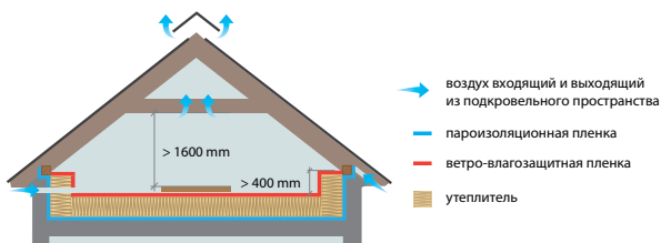
Рис. 4.10. Устройство вентиляции холодного чердака
