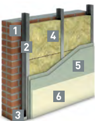
Рис. 6.7. Система ТН-СТЕНА Стандарт
