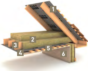
Рис. 4.9. Система ТН-ПОЛ Чердак
