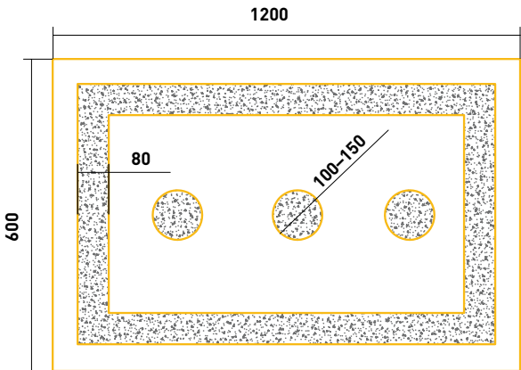
Рис. 7.23. Схема нанесения клея контурно-маячковым способом
