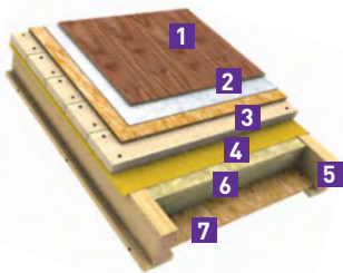
Рис. 5.1. Система ТН-ПОЛ Лайт
