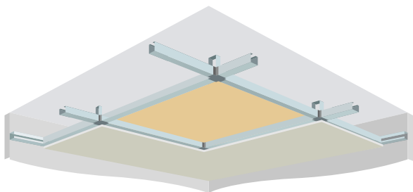
Рис. 5.18. Обшивка листами ГКЛ
