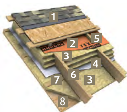
Рис. 4.1. Система ТН-ШИНГЛАС Мансарда
