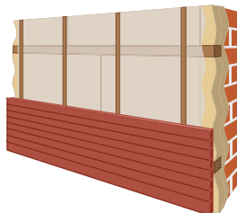
Рис. 7.6. Монтаж сайдинга
