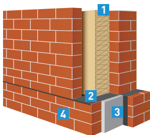
Рис. 7.11. Гидроизоляционная отсечка
