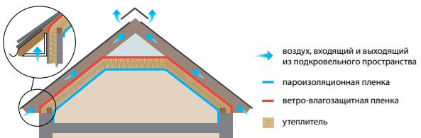
Рис. 4.2. Устройство вентиляции мансарды
