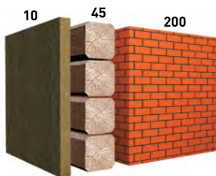
Рис. 1.1. Сравнение материалов при одинаковой теплосберегающей способности
