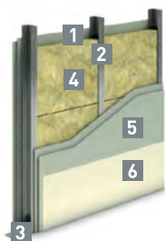
Рис. 6.1. Система ТН-СТЕНА Акустик
