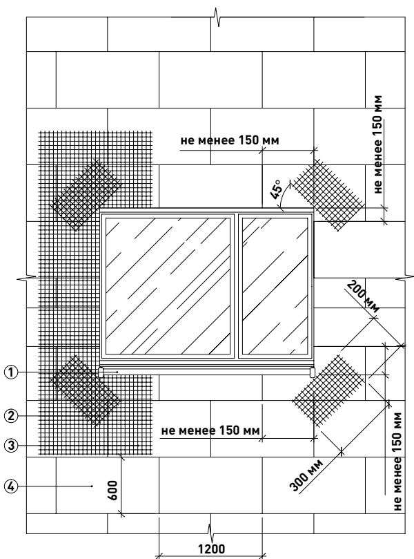
Рис. 7.28. Процесс усиления угла проема элементом из стеклотсетки
