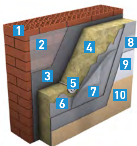
Рис. 7.18. Система ТН-ФАСАД Декор
