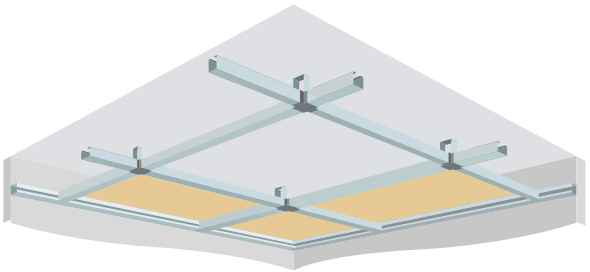
Рис. 5.17. Укладка плит ТЕХНОАКУСТИК
