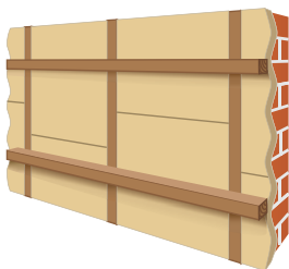
Рис. 7.4. Установка горизонтального каркаса
