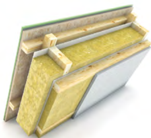
Рис. 4.8. Устройство мансарды
