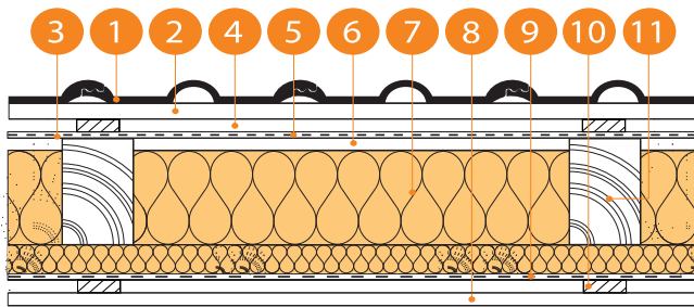
Рисунок 7. Кровля с организацией дополнительного воздушного зазора, Вариант 3
