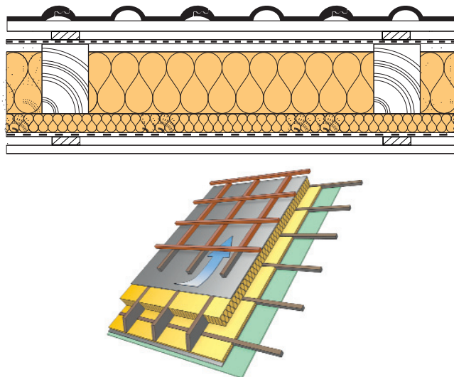
Рисунок 8. Устройство дополнительного слоя теплоизоляции с внутренней стороны
