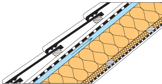
Рисунок 2. Утепление скатной кровли с организацией воздушного зазора
