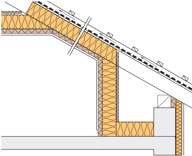
Рисунок 3. Схема устройства теплового контура скатной кровли
