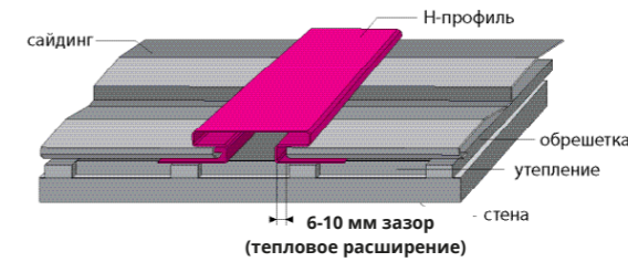
Стык с использованием H-профиля
